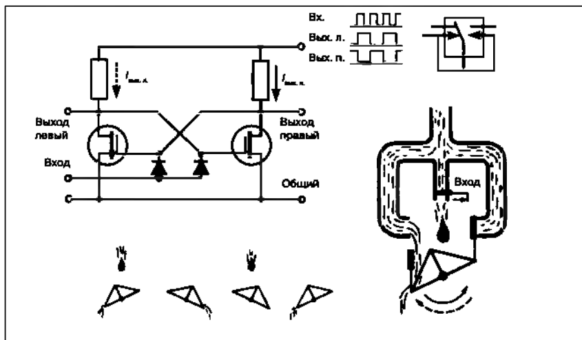
Fig. 6. FLIP-FLOP
